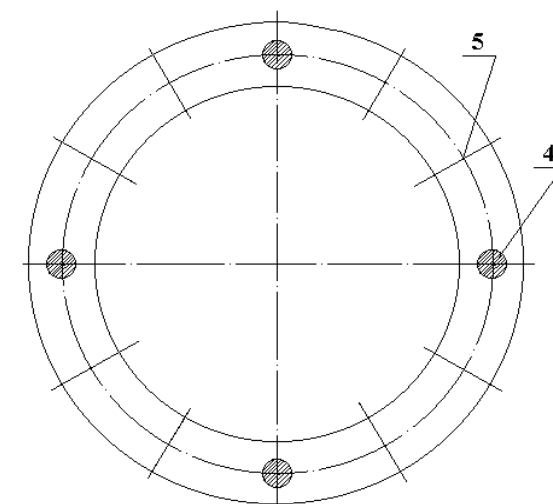
Рисунок 1 – Сопряжение гибкого колеса со ступицей выходного вала редуктора: 1 – гибкое колесо; 2 – болт; 3 – упругая втулка; 4 – отверстия с тензометрическими болтами и втулками; 5 – свободные отверстия; 6, 7 – тензорезисторы; 8 – ступица выходного вала
