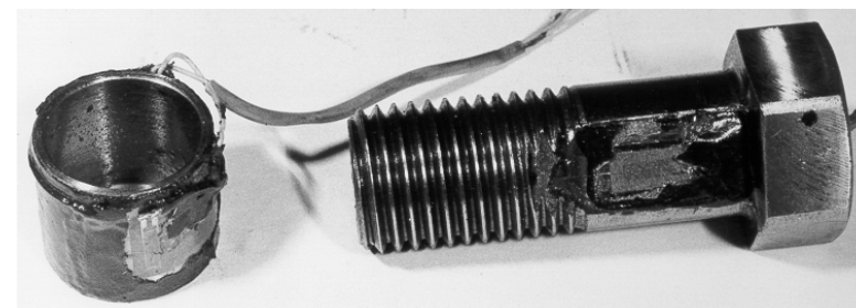
Рисунок 2 – Болт и упругая втулка с изоляцией тензорезисторов маслястойким покрытием
