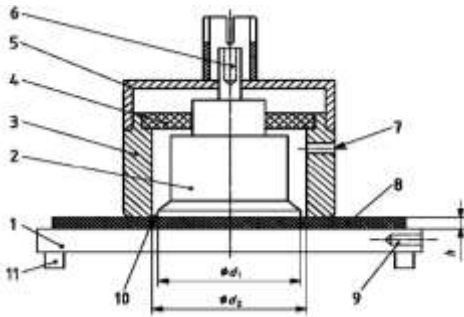
Рисунок 3 – Цилиндрический дисковый электрод с защитным кольцом ( d_1=50\text{мм} d_2=60\text{мм} ) [3]
