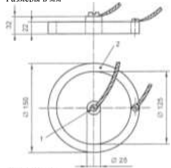
Рисунок 2 – Электроды [2]
