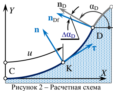
Рисунок 2 – Расчетная схема
