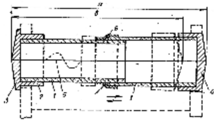
Рис. 1. Схема запобіжника з плавким елементом, виконаним з матеріалу, що володіє ефектом "пам'яті форми"
