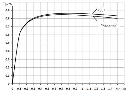
Рис. 7. Зависимости \eta = f(M_C) для двух модификаций ВДПМ
