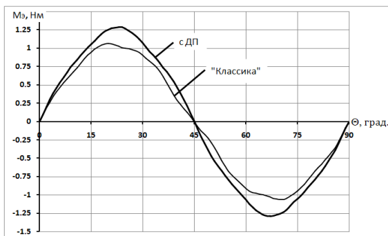
Рис. 5. Зависимости M_{\Theta} = f(\Theta)
