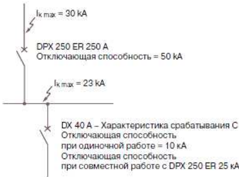
Рис. 16 – Координація роботи вимикачів Legrand.
