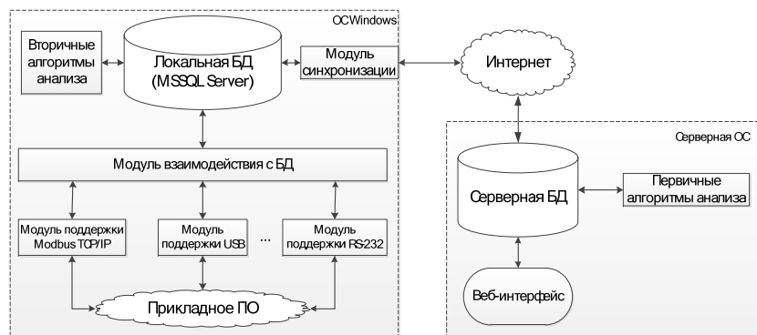
Рис. 2 – Программная архитектура системы
