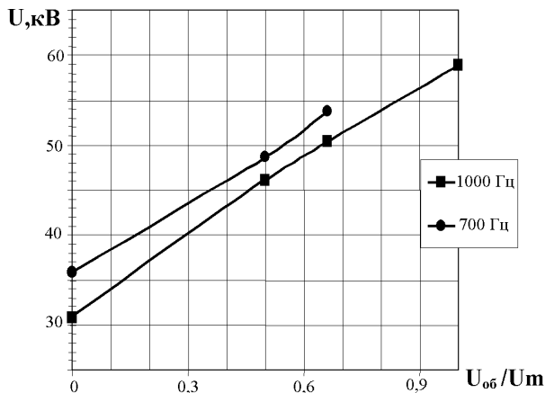
Рисунок 6 – Зависимость предпробивного напряжения электродной системы от относительной амплитуды обостренного импульса напряжения
