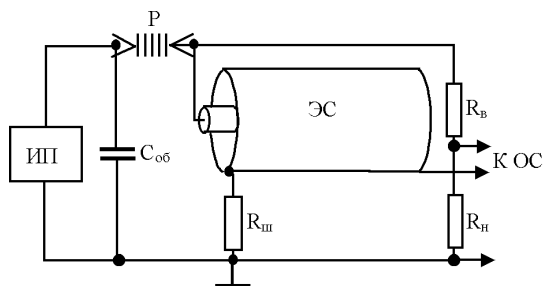
Рисунок 1 – Высоковольтный источник питания: И.п. – источник питания, C_{об} – обостряющая емкость, P – многозазорный искровой разрядник, ЭС – электродная система, R_{ш} – токовый шунт, R_{н} – низковольтное, плечо делителя напряжения, R_{в} – высоковольтное плечо делителя напряжения, ОС – осциллограф
