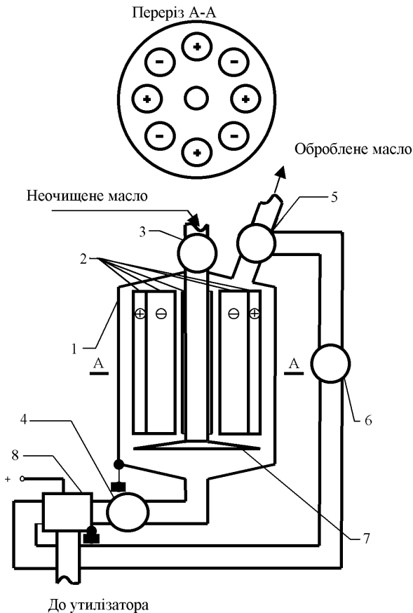
Рисунок 4 – Схема електрофізичного способу фільтрації трансформаторного масла: 1 – корпус, 2 – електроди, 3,4 – кран, 5 – кран реверсний, 6 – насос, 7 – відбивач-розпорошувач сітчастий, 8 – коагулятор
