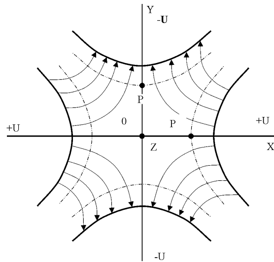
Рисунок 1 – Електричне поле квадрупольної системи електродів
