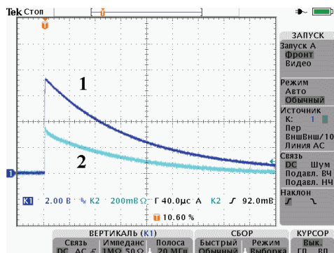
Рисунок 15 – Осцилограми спадної частини імпульсу напруги між електродами СЛ-48
