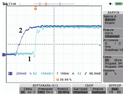
Рисунок 12 – Осцилограмми фронтової частини імпульсу напруги між електродами СЛ-48 при тиску у високовольтному комутаторі p = 6,5 атм., зарядній напрузі Еталону-СН U = 5 кВ і смузі пропускання осцилографа 20 МГц
