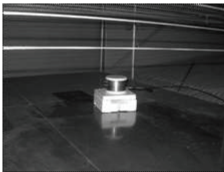
Рисунок 9 – Установка вимірювального перетворювача СПЕФВ-ЕО між електродами СЛ-48 (фотоприймач вимірювача й осцилограф розташовано у вимірювальній кабіні)
