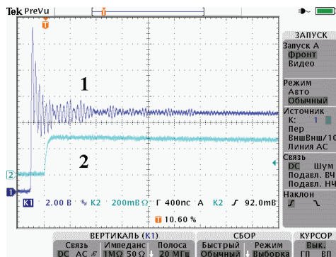
Рисунок 17 – Осцилограми фронтної частини імпульсу напруги між електродами СЛ-48 при тиску у високовольтному комутаторі p = 2,5 атм., зарядній напрузі Еталону-СН U = 5 кВ, смузі пропускання осцилографа 20 МГц і ввімкнені на виході ОДН-20 інтегруючого ланцюжка з недостатньою постійною інтегрування
