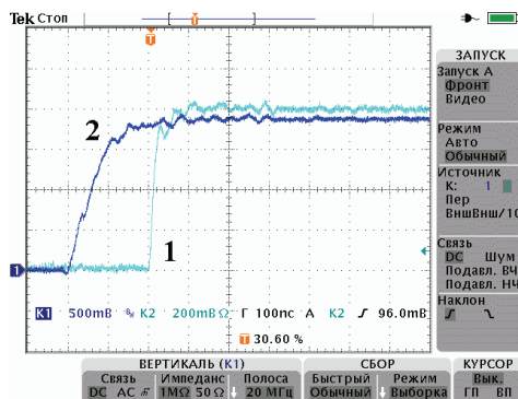
Рисунок 14 – Осцилограми фронтової частини імпульсу напруги між електродами СЛ-48 при тиску у високовольному комутаторі p = 6,5 атм., зарядній напрузі Еталону-СН U = 20 кВ і смузі пропускання осцилографа 20 МГц
