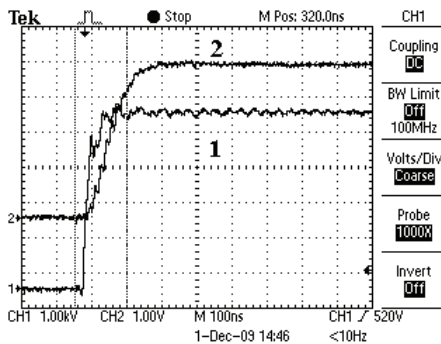
Рисунок 26 – Осцилограми фронтвої частини імпульсу напруги між електродами СЛ-48 при тиску у високовольтному комутаторі p = 6,5 атм., зарядній напрузі Еталону-СН U = 5 кВ, смузі пропускання осцилографа 100 МГц і ввімкнені на виході СДН-10 інтегруючого ланцюжка з достатньою постійною інтегрування
