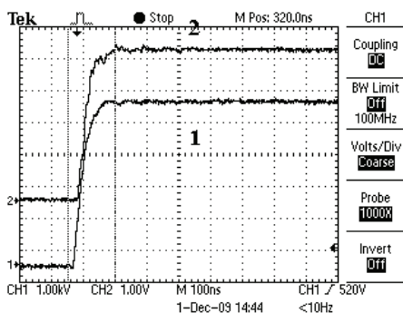
Рисунок 23 – Осцилограми фронтівій частини імпульсу напруги між електродами СЛ-48 при тиску у високовольтному комутаторі p = 0 атм., зарядній напругі Еталону-СН U = 5 кВ і смузі пропускання осцилографа 100 МГц
