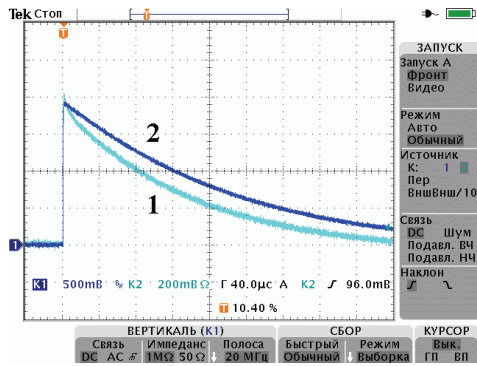
Рисунок 10 – Осцилограмми спадної частини імпульсу напруги між електродами СЛ-48
