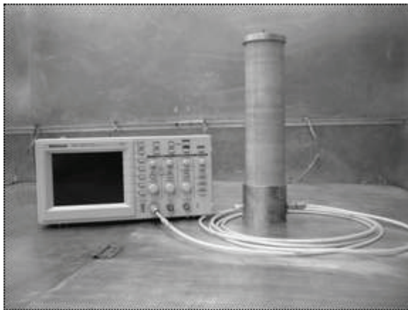
Рисунок 2 – Загальний вид омичного дільника імпульсів високої напруги ОДН-6
