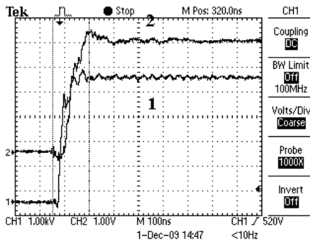
Рисунок 25 – Осцилограми фронтвої частини імпульсу напруги між електродами СЛ-48 при тиску у високовольтному комутаторі p = 6,5 атм., зарядній напрузі Еталону-СН U = 5 кВ, смузі пропускання осцилографа 100 МГц і ввімкнені на виході СДН-10 інтегруючого ланцюжка з недостатньою постійною інтегрування
