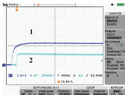
Рисунок 19 – Осцилограми фронтної частини імпульсу напруги між електродами СЛ-48 при тиску у високовольтному комутаторі p = 2,5 атм., зарядній напрузі Еталону-СН U = 20 кВ, смузі пропускання осцилографа 20 МГц і ввімкненні на виході ОДН-20 інтегруючого ланцюжка з зайвою постійною інтегрування
