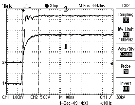
Рисунок 21 – Осцилограми фронтової частини імпульсу напруги між електродами СЛ-48 при тиску у високовольтному комутаторі p = 2,5 атм., зарядній напрузі Еталону-СН U = 5 кВ і смузі пропускання осцилографа 100 МГц
