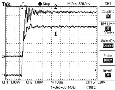
Рисунок 24 – Осцилограми фронтвої частини імпульсу напруги між електродами СЛ-48 при тиску у високовольтному комутаторі p = 6,5 атм., зарядній напрузі Еталону-СН U = 5 кВ і смузі пропускання осцилографа 100 МГц
