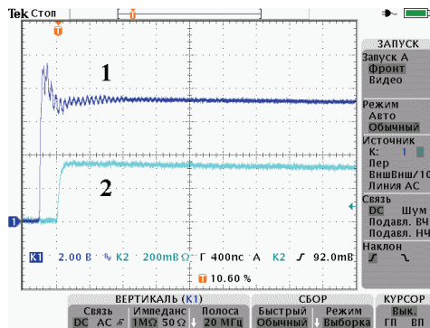
Рисунок 18 – Осцилограми фронтної частини імпульсу напруги між електродами СЛ-48 при тиску у високовольтному комутаторі p = 2,5 атм., зарядній напрузі Еталону-СН U = 5 кВ, смузі пропускання осцилографа 20 МГц і ввімкнені на виході ОДН-20 інтегруючого ланцюжка з достатньою постійною інтегрування
