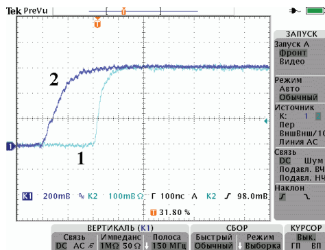
Рисунок 13 – Осцилограми фронтової частини імпульсу напруги між електродами СЛ-48 при тиску у високовольному комутаторі p = 0 атм., зарядній напрузі Еталону-СН U = 5 кВ, смузі пропускання осцилографа 150 МГц і ввімкнені на виході ОДН-300 інтегруючого ланцюжка
