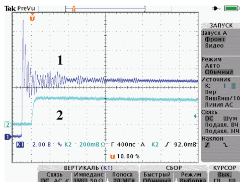
Рисунок 16 – Осцилограми фронтної частини імпульсу напруги між електродами СЛ-48 при тиску у високовольтному комутаторі p = 2,5 атм., зарядній напрузі Еталону-СН U = 5 кВ і смузі пропускання осцилографа 20 МГц
