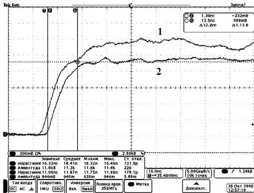
Рисунок 1 – Осцилограми фронту імпульсу напруги з виходу шупа високовольтного P6015A (1) і фронту імпульсу напруги з виходу вимірювача СПЕФВ-ЕК (2) при U_{зар} = 10 кВ
