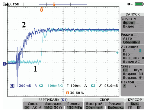
Рисунок 11 – Осцилограмми фронтової частини імпульсу напруги між електродами СЛ-48 при тиску у високовольтному комутаторі p = 0 атм., зарядній напрузі Еталону-СН U = 5 кВ і смузі пропускання осцилографа 150 МГц
