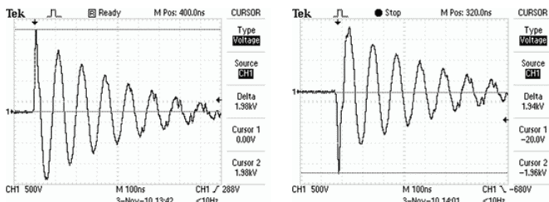
Рисунок 7 – Типовые осциллограммы испытательного напряжения 5 уровня положительной и отрицательной полярностей
