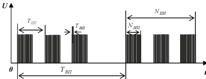
Рисунок 2 – Циклограмма многоразовых всплесков
