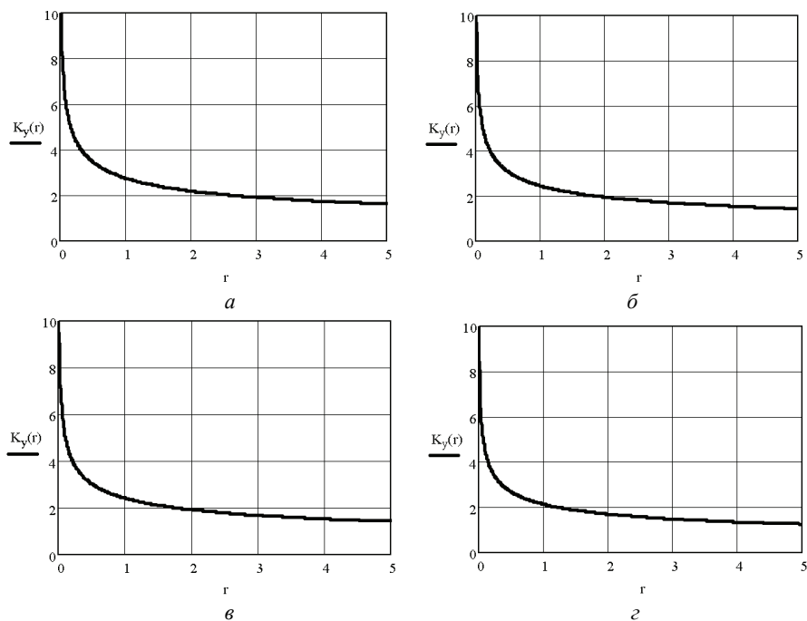
Рисунок 3 – Зависимости коэффициента усиления электрического поля в жидком ди- электрике от расстояния до острого края обкладки для пленочных диэлектрических систем: а – полиэтилентерефталатная система, пропитанная трансформаторным мас- лом Т-1500; б – комбинированная полипропиленово-полиэтилентерефталатная систе- ма, пропитанная трансформаторным маслом Т-1500; в – полиэтилентерефталатная систе- ма, пропитанная полиметилсилоксановой жидкостью ПМС-20; г – комбинированная полипропиленово-полиэтилентерефталатная система, пропитанная полиметилсилокса- новой жидкостью ПМС-20
