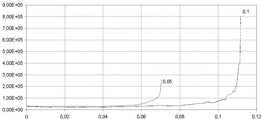
Рисунок 11 – Изменение напряженности поля в зависимости от изменения остроты стержня
