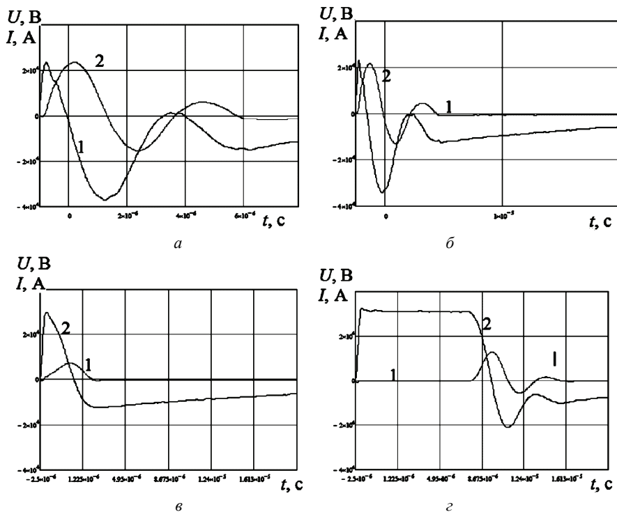
Рисунок 2 – Осциллограммы обработки порошка Ti в режиме №2: 1 – U(t) ; 2 – I(t) ; а – 200 разрядов из 4000 разрядов; б – 2000 разрядов из 4000 разрядов; в – 3235 разрядов из 4000 разрядов; з – 3800 разрядов из 4000 разрядов
