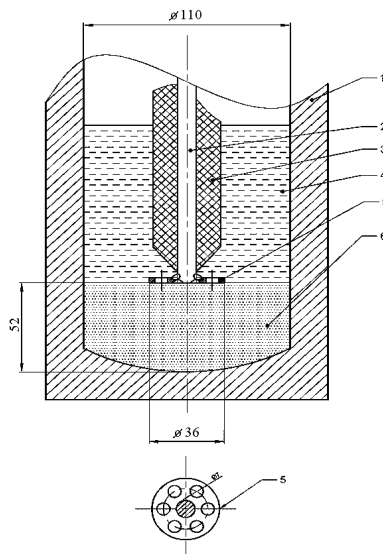
Рисунок 1 – Схема воздействия: 1 – разрядная камера; 2 – токовод; 3 – проходной изолятор; 4 – керосин; 5 – металлическая розетка; 6 – обрабатываемый порошок Ti
