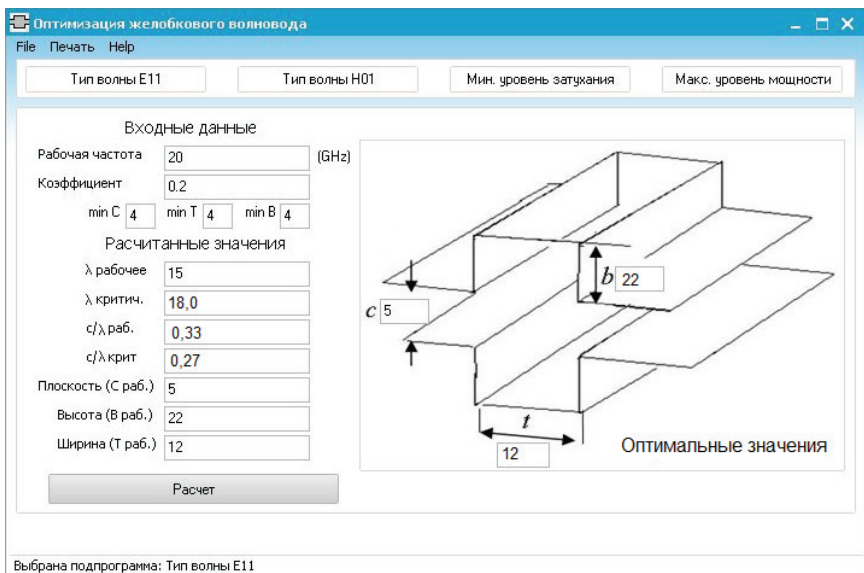
Рисунок 7 – Геометрия желобкового хвилеводу відповідна до робочої частоти хвилі E_{11}
