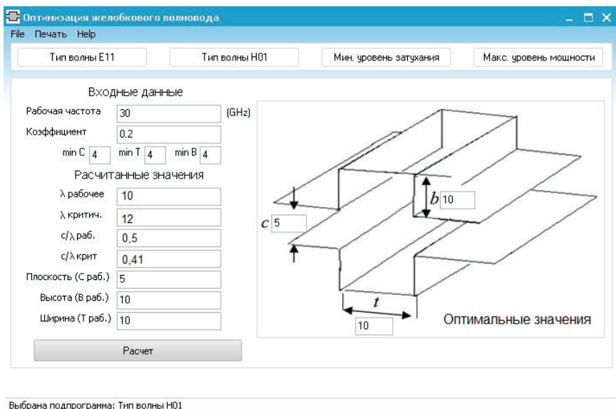
Рисунок 8 – Геометрия желобкового хвилеводу відповідна до робочої частоти хвилі H_{01}
