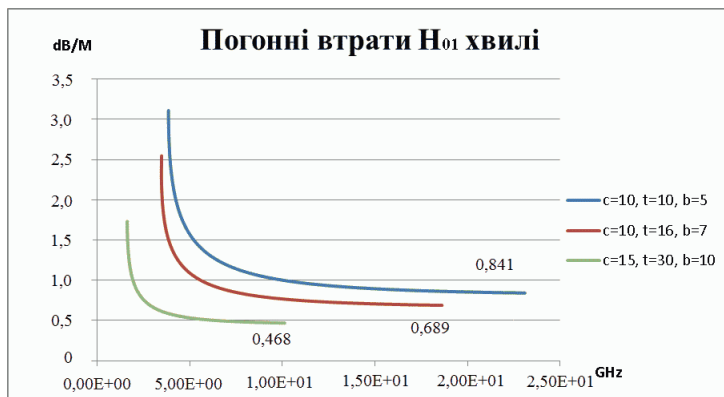
Рисунок 3 – Залежність рівня згасання хвилі N_{01} від геометрії жолобкового хвильоводу
