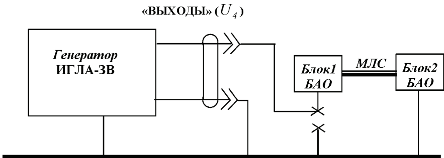
Рисунок 7 – Схема испытаний БАО в режиме « U_4 »
