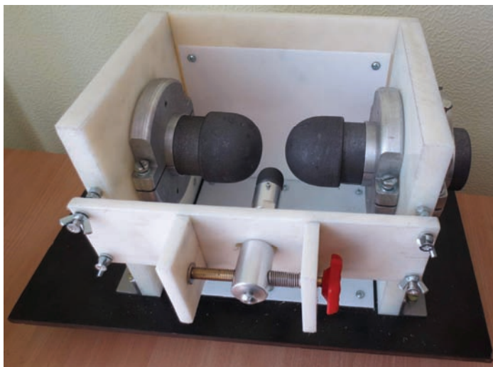
Рисунок 1 – Общий вид высоковольтного управляемого разрядника с графитовыми электродами РВГУ-50
