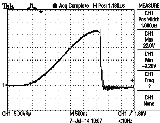
Рисунок 5- осциллограмма импульса напряжения поджига U_n с пробоем промежутка «с» = 10 мм между основным и поджигающим электродами (основной электрод соединен с R_{разр.} ); «а»=10
