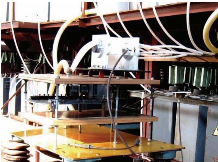
Рисунок 6 – Внешний вид рабочего стола генератора тока молнии ГИТМ-10/350 с установленным на нем разрядником РВГУ-50
