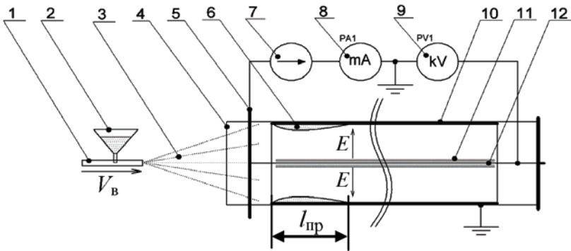
Рисунок 1 – Стенд для определения эффективности электрической фильтрации: 1 – смеситель; 2 – бункер подачи пыли; 3 – воздушно-пылевой поток; 4 – корпус макета ЭС ЭФ; 5 – шпилька натяжения КЭ; 6 – пыль, осевшая на ОЭ; 7 – источник высокого напряжения; 8 – миллиамперметр; 9 – киловольтметр; 10 – ОЭ; 11 – свечение коронного разряда; 12 – КЭ
