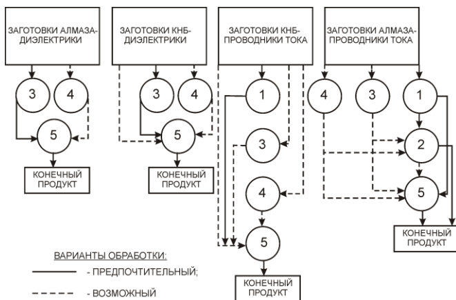
Рисунок 4 – К методологии реализации потенциала различных методов формообразования лезвийных инструментов из ПСТМ
