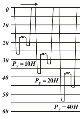
Рис. 2 – Глубина внедрения (в мкм) алмазного конуса 2\gamma=120^\circ в армо-железо ( 103\text{ HV} ) при вдавливании, царапании и остановках
