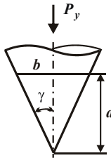
Рис. 1 – Расчетная схема площади поперечного сечения среза
