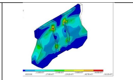
Рис. 4 – 5 собственная форма колебаний
