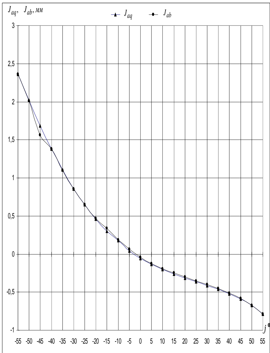
Рис. 9. Зазоры у вершин зубьев гибкого и жесткого колес волновой передачи редуктора механизма поворота передвижного миксера МП – 600АС при нагрузке 5 \times 10^5 \text{ Н} \cdot \text{м}
