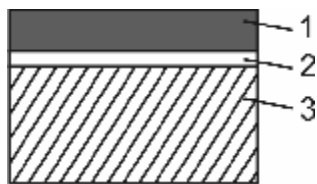
Рис. 1. Схема оксидного кобальт-титанового анода:
