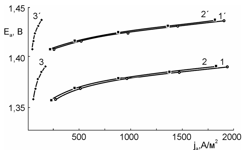
Рис. 2. Суммарные (1, 1'), парциальные выделения хлора (2, 2') и кислорода (3, 3') поляризационные кривые на ОРТА (1 – 3) и \text{Co}_3\text{O}_4/\text{TiO}_2 -покрытии (1' – 3') в 2\text{M NaCl} при 293 \text{ K} .
