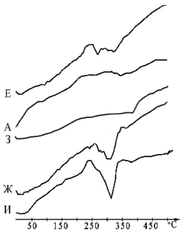
Рис. 2. Деривато-граммы некоторых образцов (ДТА-кривые)
