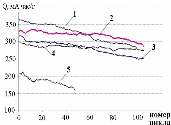
Рисунок – Зависимость удельной емкости от количества заряд-разрядных циклов в режиме C/15 для графитов различных марок: 1 – LBG-73; 2 – ГЛ-1Б; 3 – ЭУЗМ; 4 – ГЛ-1А; 5 – ГЛ-1.
