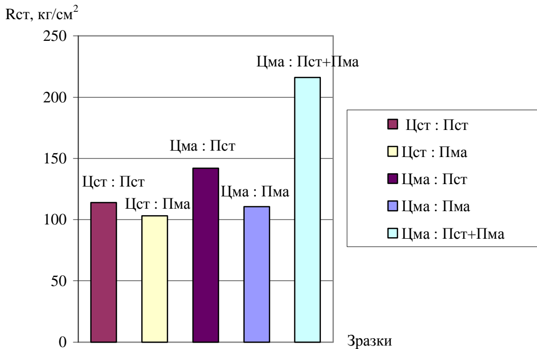
Рис. 1. Діаграма міцності зразків на одноосьовий стиск залежно від механоактивації вихідних компонентів (“ст” – стандартні і “ма” – механоактивовані цемент й пісок)
