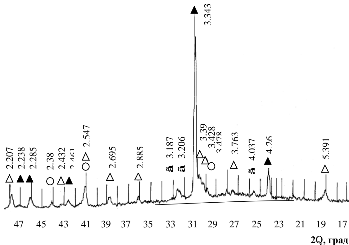
р – кварц; r – муліт; š – \alpha - \text{Al}_2\text{O}_3 ; ã – кристобаліт Рис. 3. Рентгенограма зразка, випаленого при температурі 1150 °С
