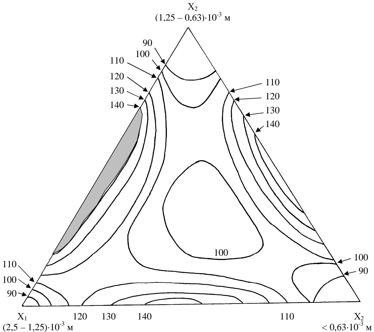
Рисунок – Діаграма «склад – межа міцності при стиску» зразків шлаколузних бетонів, отриманих з використанням гранвідсіву
