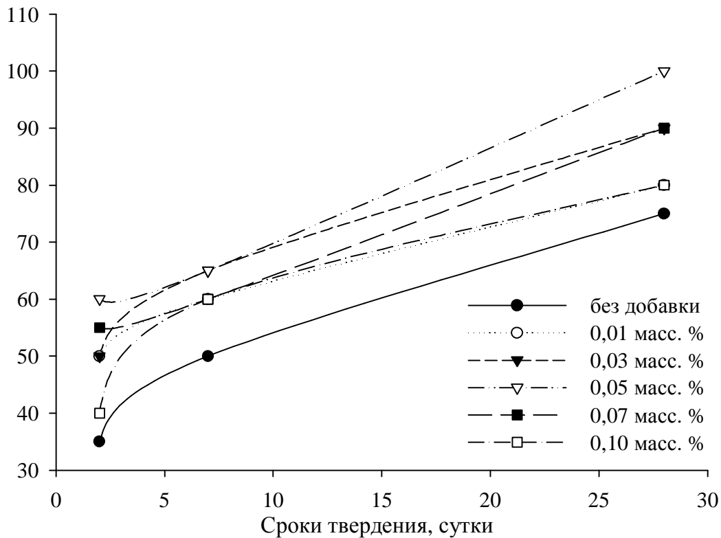
Рис. 6. Зависимость предела прочности при сжатии от срока твердения для цемента с добавкой НСАКМА
