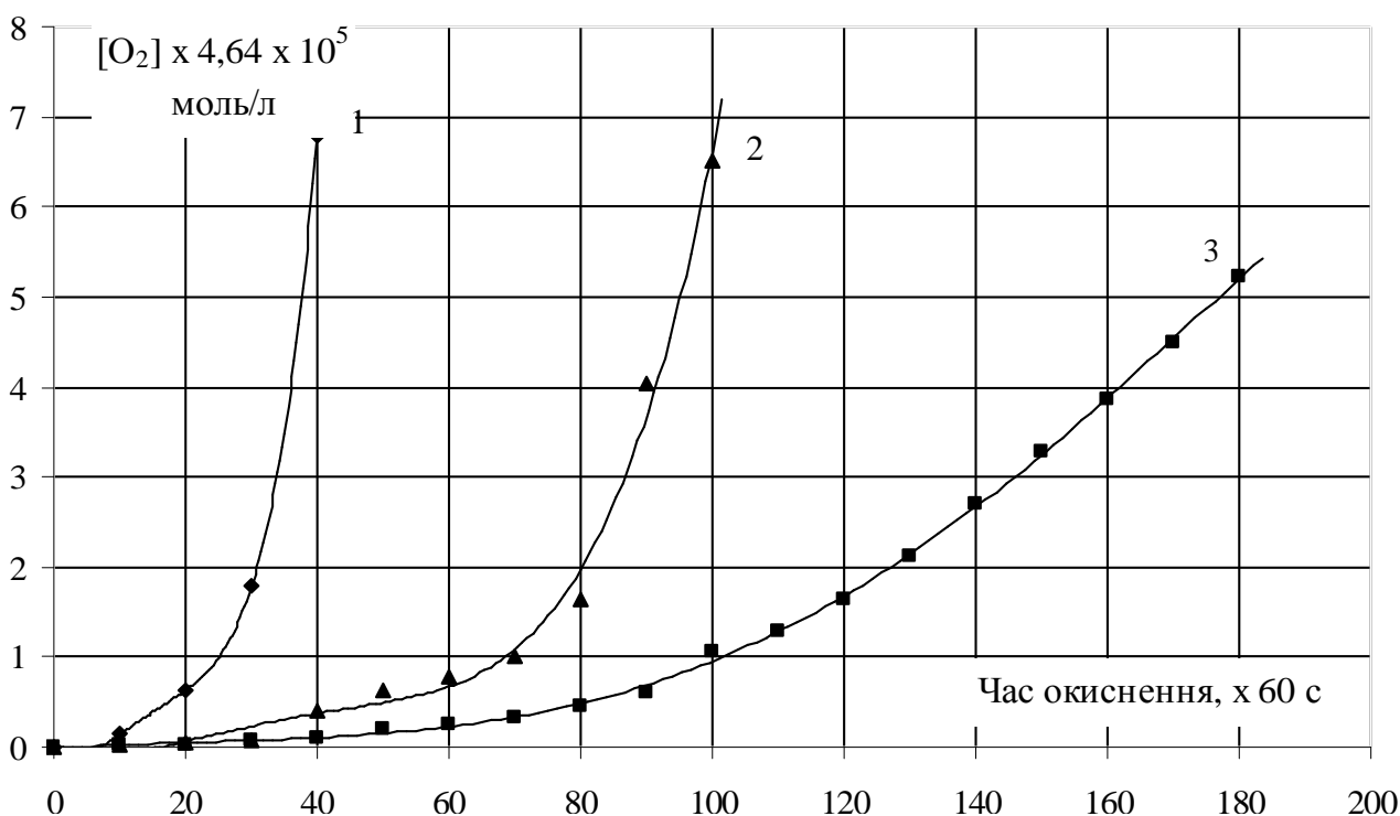
Рис. 1. Крива поглинання кисню в дослідних зразках глазури:
