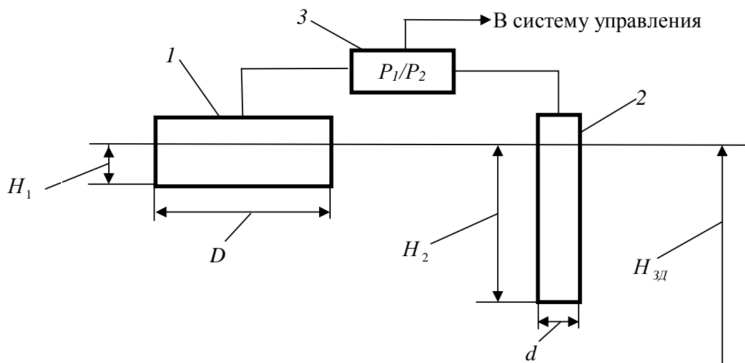
Рис. 2 – Регулятор уровня: 1 – поплавок с меньшей высотой и большей плотностью поперечного сечения S_1 = \kappa D^2 ; 2 – поплавок с большей высотой и меньшей площадью поперечного сечения S_2 = \kappa d^2 ; 3 – блок соотношения P_1/P_2 с унифицированным выходным сигналом.
