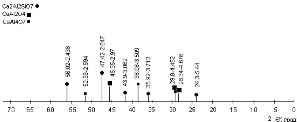
Рис. 2 – Штрих-рентгенограмма состава № 2
