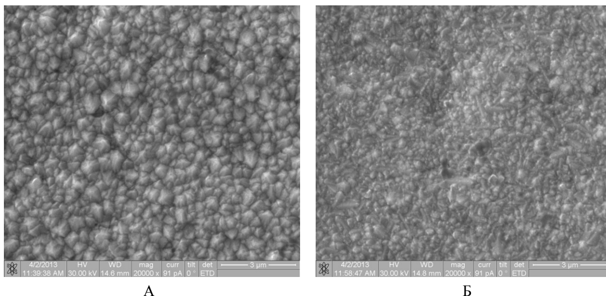
Рис. 5. Растровые электронно-микроскопические изображения медных осадков, полученных из пиррофосфатного электролита, \tau = 2,5\text{ ч} ; i = 0,3\text{ А/дм}^2 ; t = 20\text{ }^{\circ}\text{C} ; \delta = 10\text{ мкм} . А – без УНМ. Б – C_{\text{УНМ}} = 0,5\text{ г/л} .
