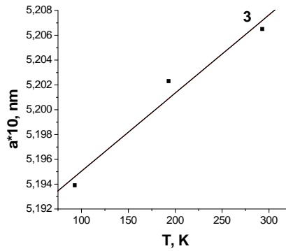
- Зависимость параметра квазикристалличности a_q от температуры
