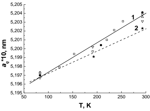
- Зависимость параметра квазикристалличности a_q от температуры
