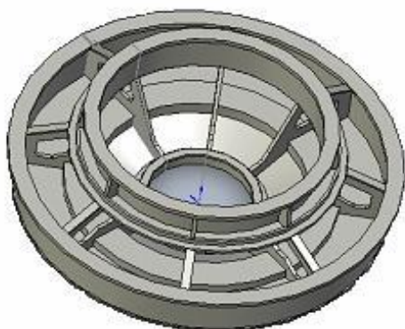
Рис. 1. Крышка гидротурбины
