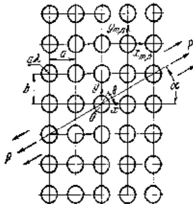
Рисунок 1-Модель двоякоперіодичних прямокутних ґрат
