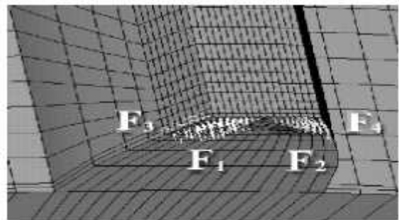
Рисунок 1 – Модель зуба довбача під робочим навантаженням
