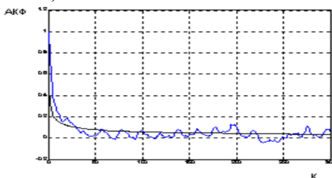
Рис.2. Автокорреляционная функция
