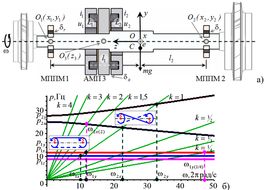
Рисунок 1. Розрахункова схема лабораторної установки ротора в МП (а) і частотна діаграма Кембелла (б)
