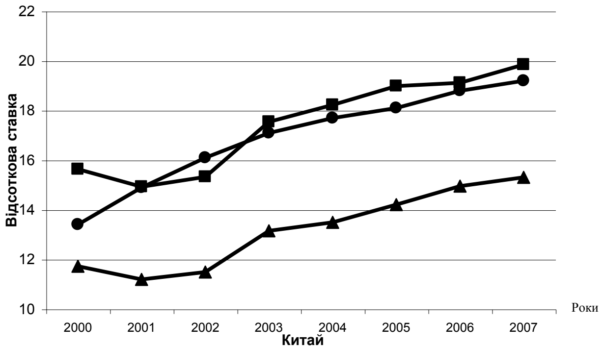
Рис. 3. Крива Лаффера для української і китайської економіки
