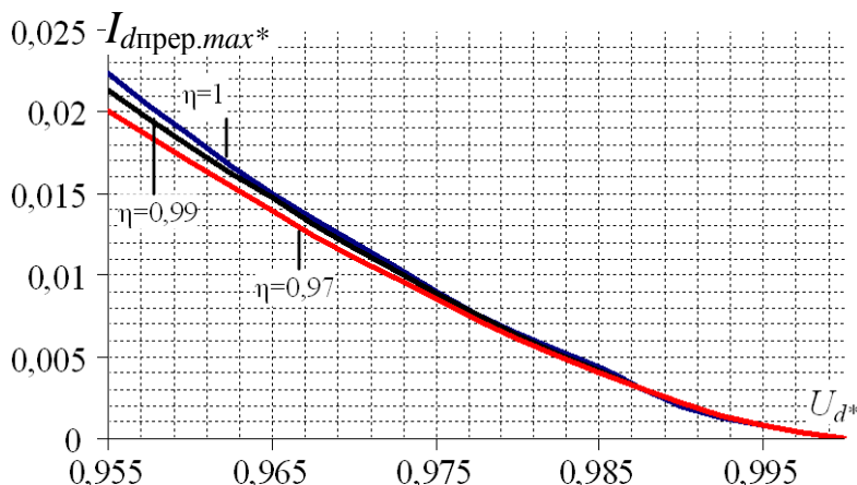
Рис. 1. Амплітуда переривчастого струму НВ з ефісним навантаженням
