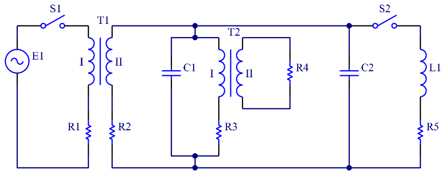
Рисунок 5 – Еквівалентна схема генеруючого тракту ЕМА товщиноміру
