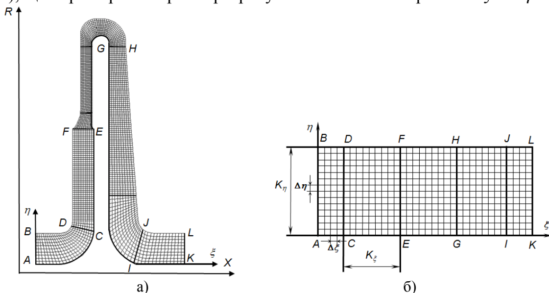
Рисунок 1 – Розрахункова область:
