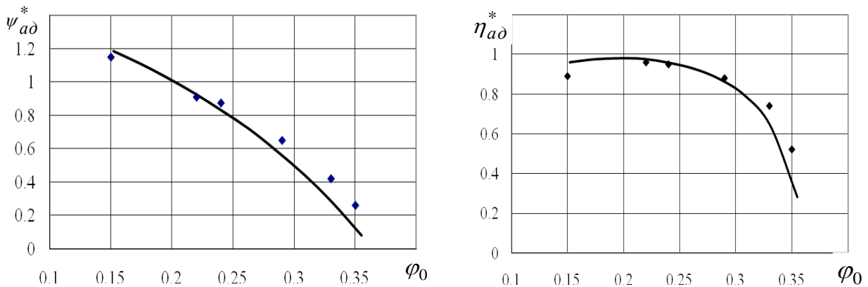
Рисунок 4 – Сумарні характеристики робочого колеса:
