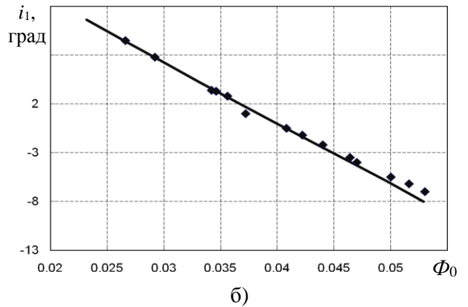
Рисунок 9 – Зіставлення результатів чисельного та експериментального досліджень у вигляді залежностей:
