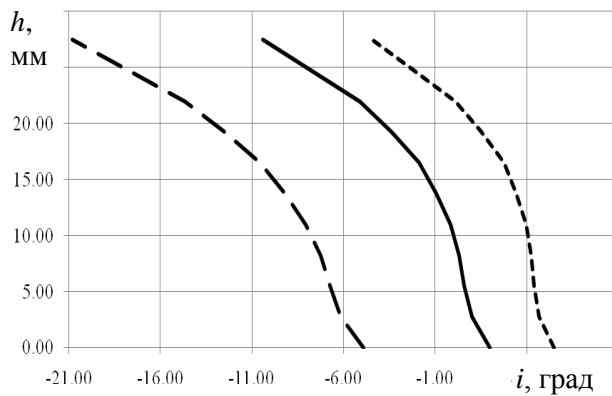
Рисунок 6 – Розподіл кутів натікання на РК по висоті проточної частини: - - - - - на режимі \varphi_0 = 0,17 ; ————— на режимі \varphi_0 = 0,22 ; - · - · - на режимі \varphi_0 = 0,33
