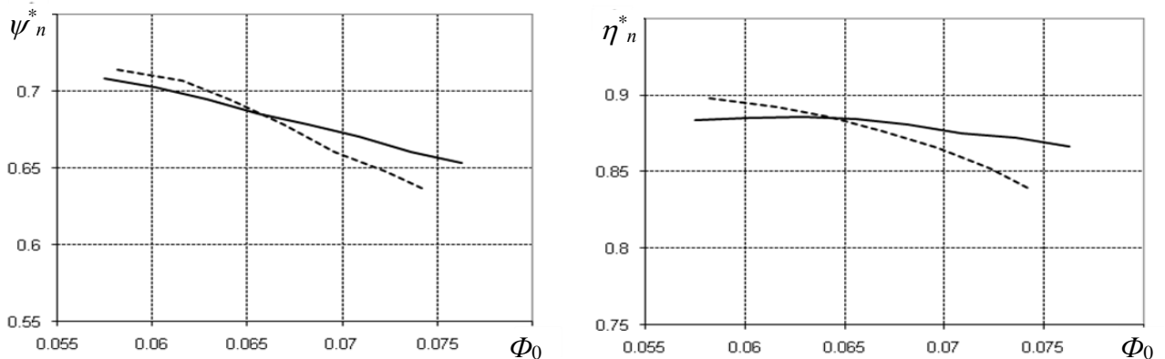
Рисунок 16 – Сумарна характеристика ступеня «Б»: — - вихідний геометричний кут \alpha_{3z} ; - - - - модифікований геометричний кут \alpha_{3z}
