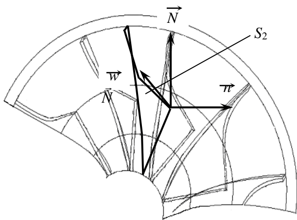
Рисунок 2 – Середина поверхня S_2
