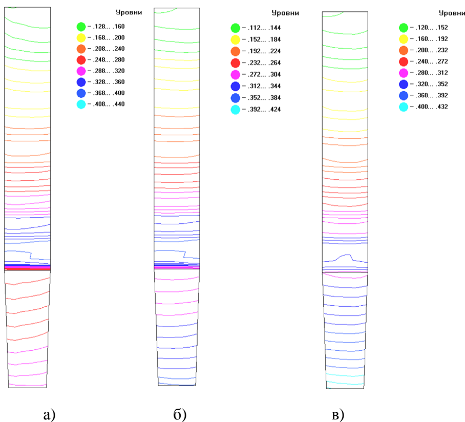
Рисунок 12 – Ізолінії чисел Маха в проточній частині щілинного і лопаткового дифузоров ступеня «А» при різних варіантах виконання лопатки РК на «розрахунковому» режимі:
