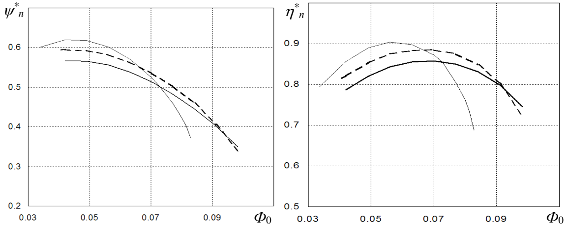
Рисунок 19 – Сумарна характеристика ступеня «В» з вихідним БЛД і двома варіантами ЛД: ——— - ступінь з БЛД; - - - - - - ступінь з ЛД в модифікованій проточній частині; ——— - ступінь з ЛД у вихідній проточній частині
