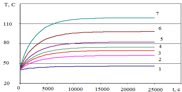
Рисунок 16 – Результати розрахунків температури ОПН при впливі першої третьої п'ятої та сьомої гармонік напруги при температурі оточуючого середовища 40 С.
