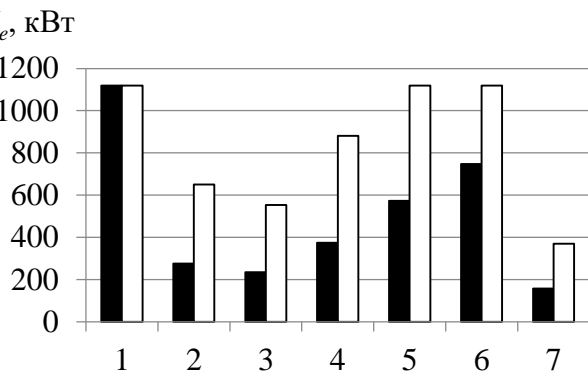
Рисунок 8 – Потужність двигуна при використанні природного газу та НГП: ■ – ГА двигуна 11ГД100М; □ – ГА двигуна 17ГД100А; 1 – Природний газ; 2 – Синтез-газ; 3 – Піролізний газ; 4 – Шахтний газ; 5 – Біогаз; 6 – Коксовий газ; 7 – Генераторний газ
