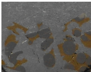
Рис.1 Микроструктура литого алюмоматричного материала с частицами композита бронза-стальная дробь.
