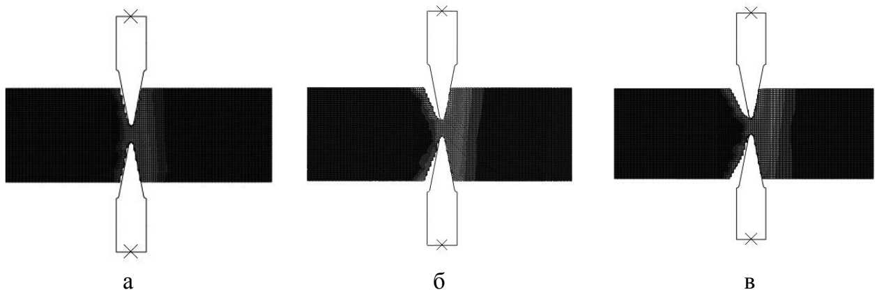
Рисунок 8 – Картина деформування (фінальна стадія) при різанні заготовок клиноподібними ножами, що рухаються по кутовому закону:
