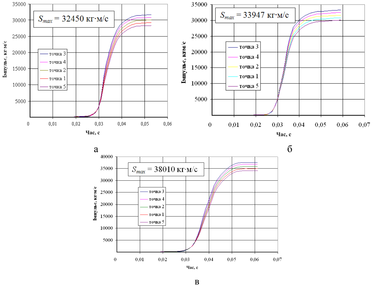
Рисунок 7 – Графіки зміни «назаднього» імпульсу для сталей:
