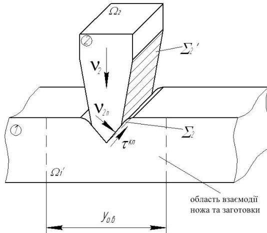
Рисунок 2 – Область контакту ножа та заготовки
