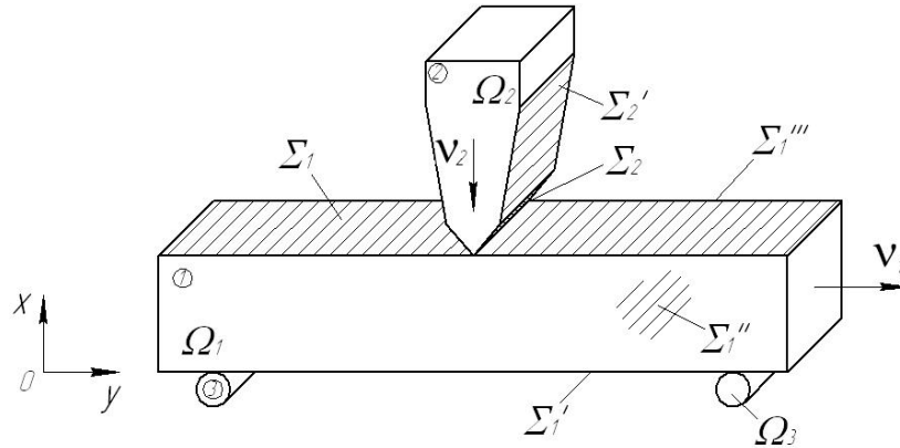
Рисунок 1 – Схема різання безперервнолитої заготовки одним ножом:
