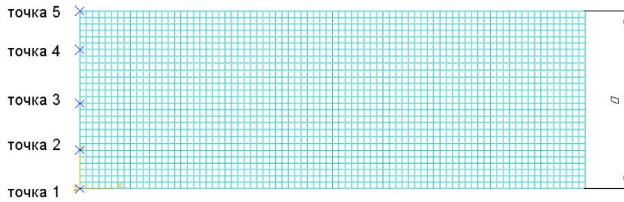
Рисунок 4 – «Контрольний переріз» з точками, у яких аналізується небажаний «назадний» імпульс
