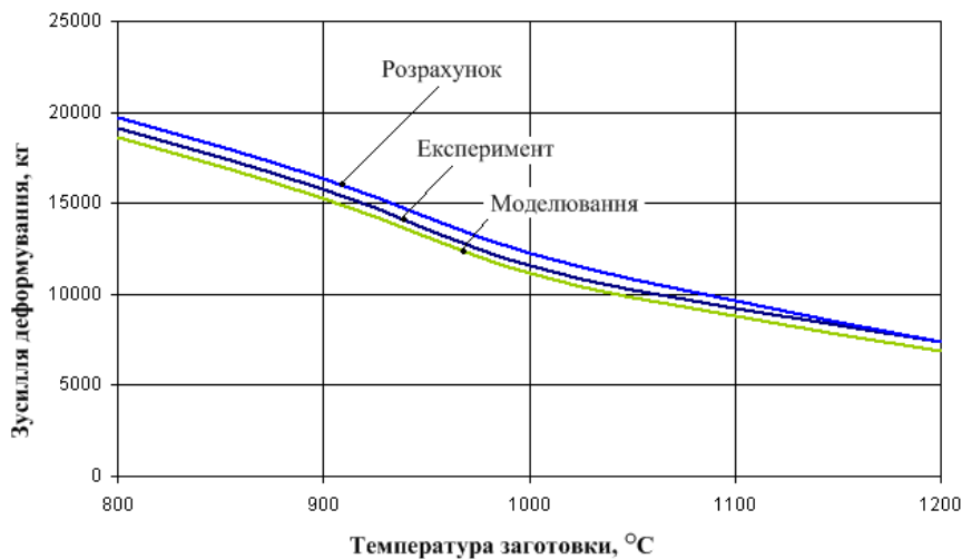
Рисунок 5 – Графіки залежності зусилля різання від температури заготовки
