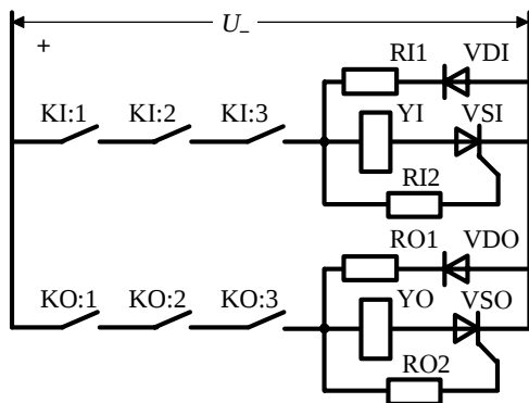
Рис. 4. Реализация шунтирования обмоток встречными диодами с помощью однооперационных тириستоров
