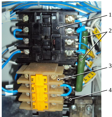
Рис. 7. Элементы коммутации силовой цепи системы управления вакуумного выключателя ВБ-4Е: 1 – контактор КИ типа ПМЛ2100; 2 – резисторы R1 R2, смонтированные на терминалах контакторов КИ и КО; 3 – блок вспомогательных контактов типа ПКЛ; 4 – контактор КО типа ПМЛ2100
