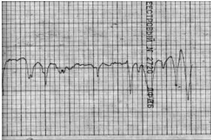
Рисунок 7 – Профилограмма обработанной деформирующим протягиванием поверхности гильзы из легированного чугуна при относительной деформации заготовки \epsilon=0,2\% .
