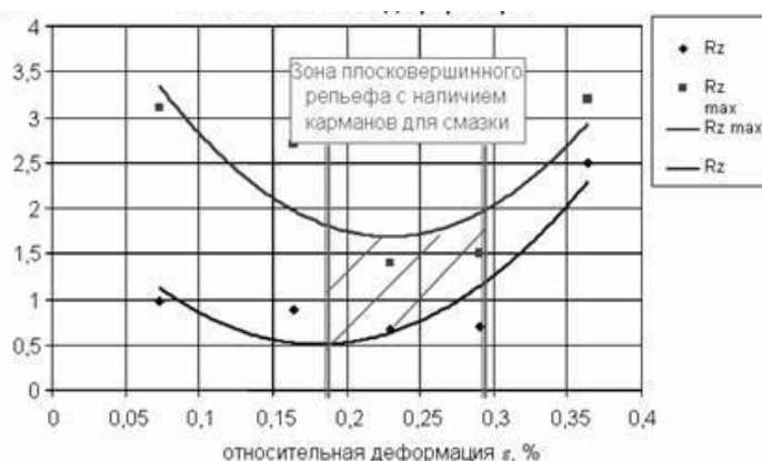
Рисунок 6 – Зависимость шероховатости протянутой поверхности от относительной деформации \varepsilon заготовки
