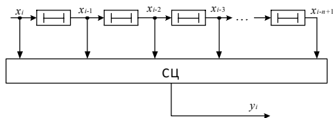
Рис. 1 – Медианный фильтр с применением сортирующей сети
