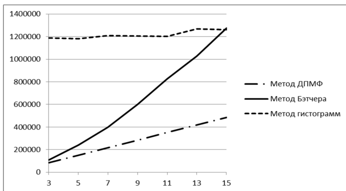
Рис. 3 - График зависимости количества циклов при фильтрации последовательности от выбранной апертуры для процессора ADSP-218x
